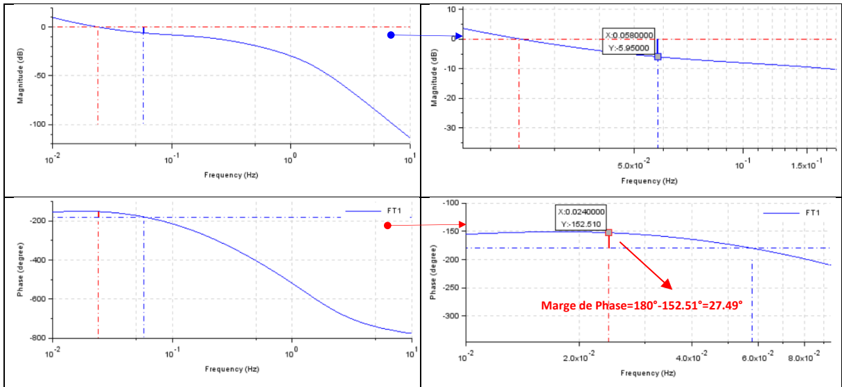
Figure 48 : Diagramme de Bode en boucle ouverte - Marges de gain et de phase – Réglage ma à +3dB
