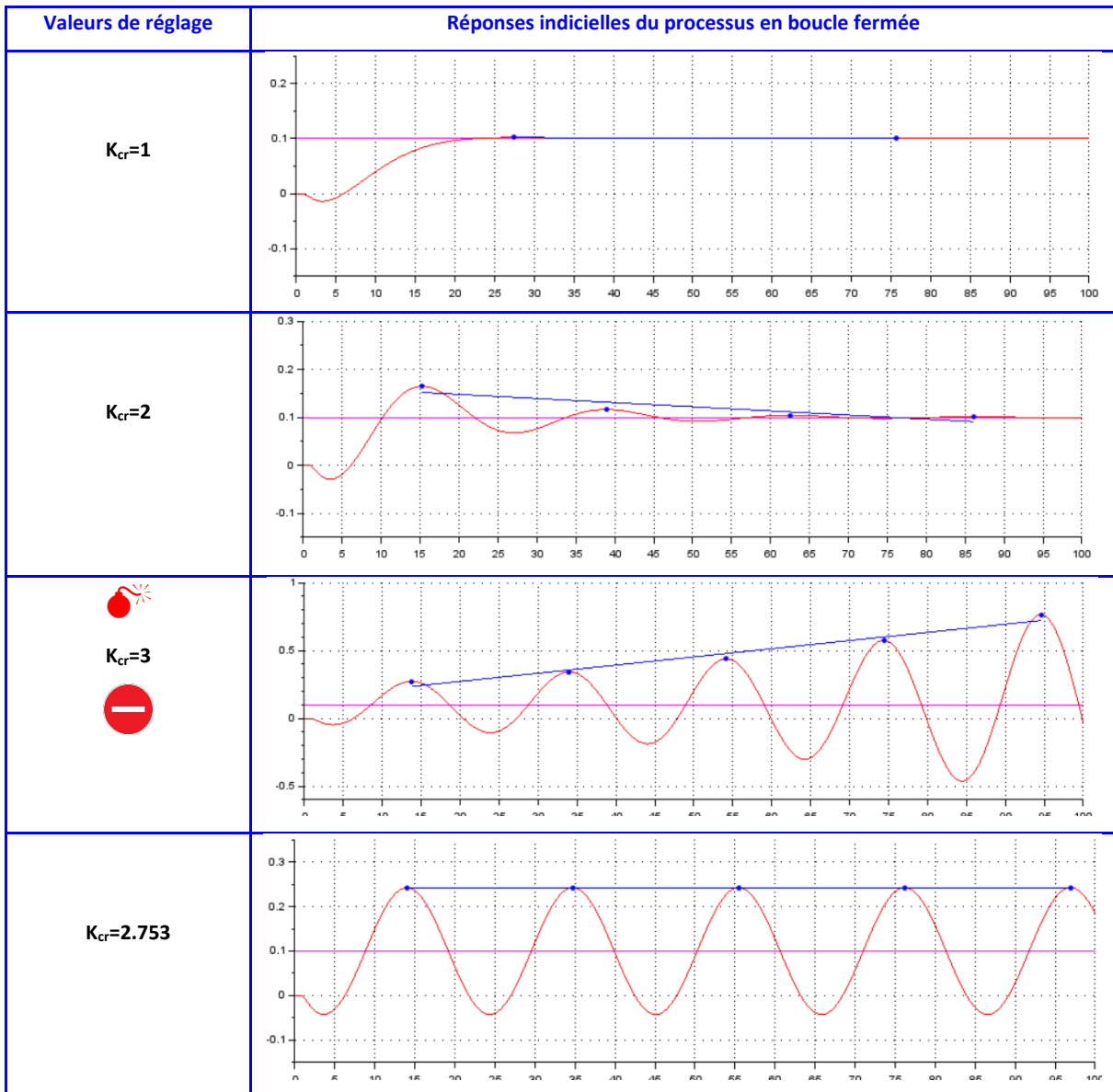
Figure 61 : Exemple de réglage du procédé de Ziegler-Nichols
