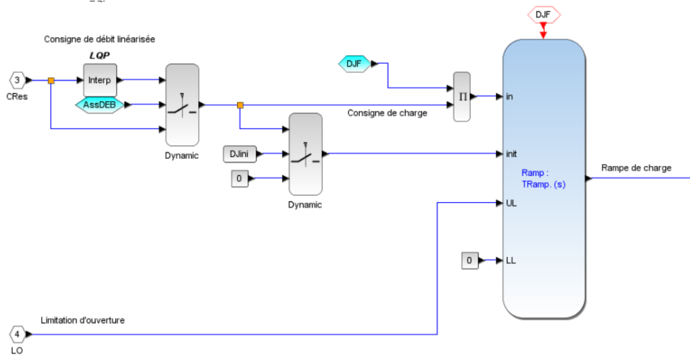
Figure 46 : Extrait du consignateur de charge dans les modèles HYDROTUR
