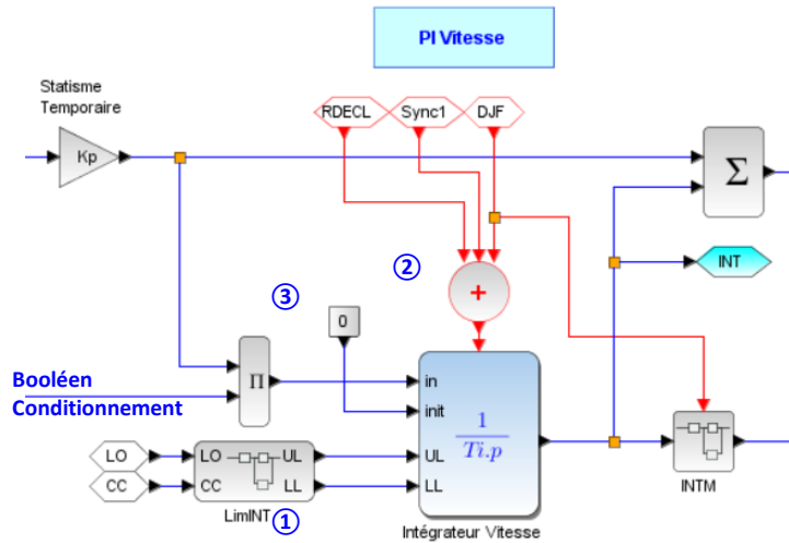
Figure 37 : Intégrateur IntLim dans le régulateur de vitesse HYDROTUR
