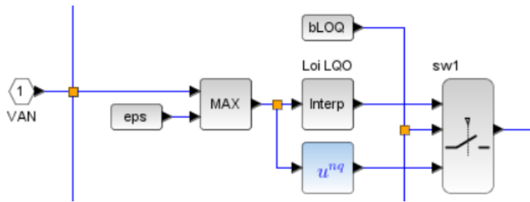
Figure 43 : Approximation de la loi Débit/Ouverture dans TURBADDUC modèle FR2
