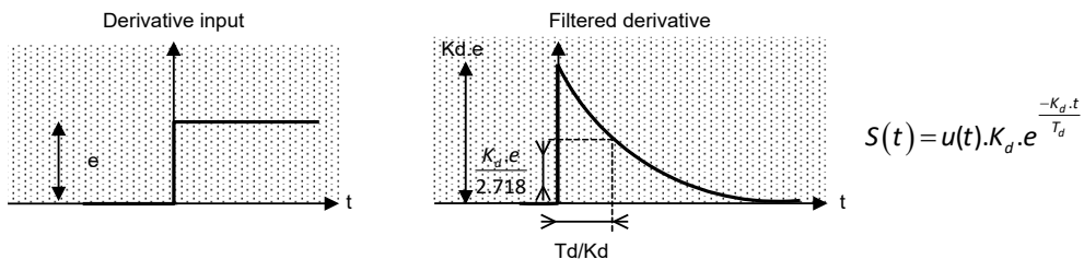
Figure 21 : Rappel de principe du dérivateur filtré
