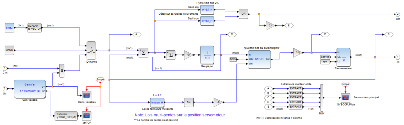
Figure 29 : Extrait des systèmes copiant SYSCOP_I des injecteurs (voir schémathèque PELTON) – Implantation multivariables
