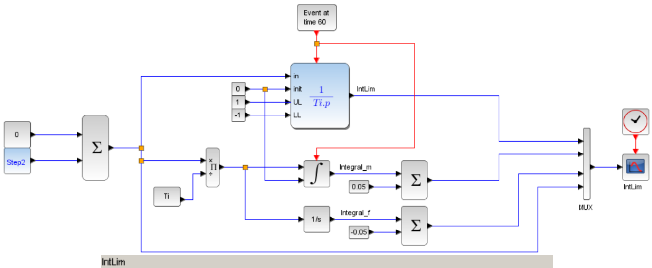
IntLim Comparaison des intégrateurs IntLim (HYDROTUR) et Integral_m, Integral_f (Scilab-Xcos)
