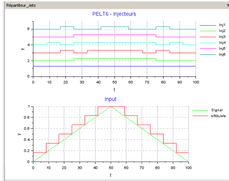
Figure 49 : Programme de test Répartiteur_Jets1.zcos
