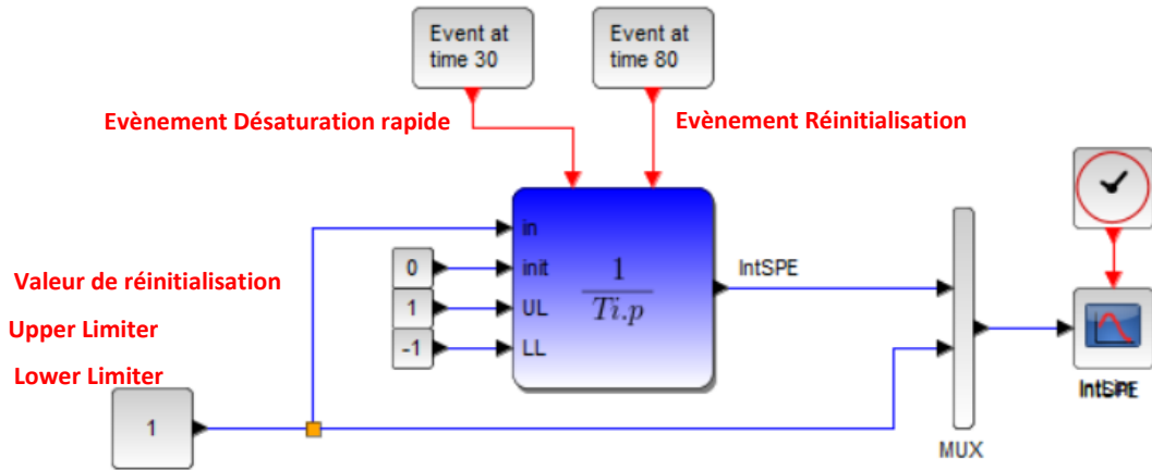
Figure 38 : Intégrateur à fuite IntSPE
