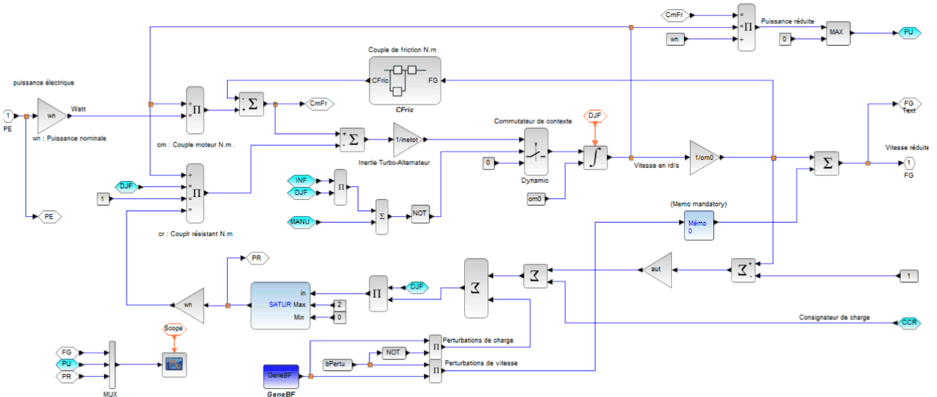
Figure 33 : Utilisation du perturbateur GeneBF dans les modules "Réseau" des simulateurs HYDROTUR
