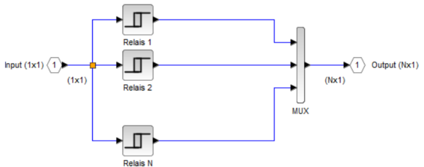
Figure 47 : Principe du composant Relais_H
