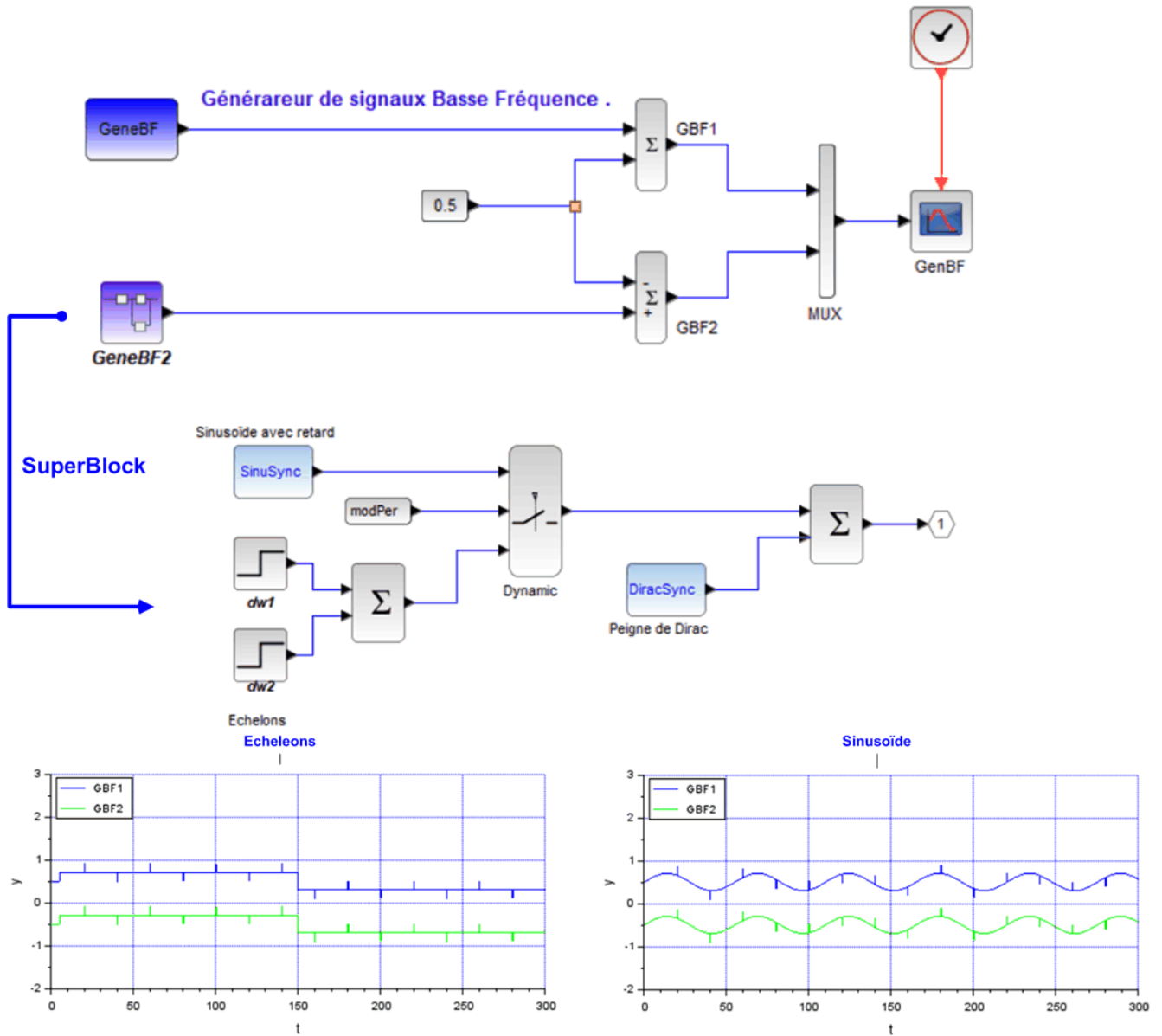
Figure 32 : Programme de test du générateur GeneBF.zcos
