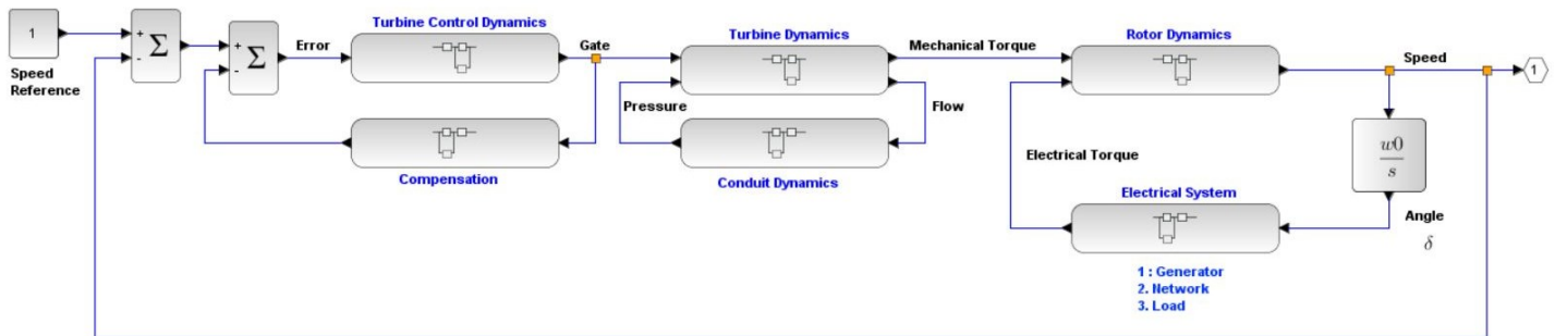
Figure 2 : Principe de base des simulateurs HYDROTUR pour turbines hydrauliques
