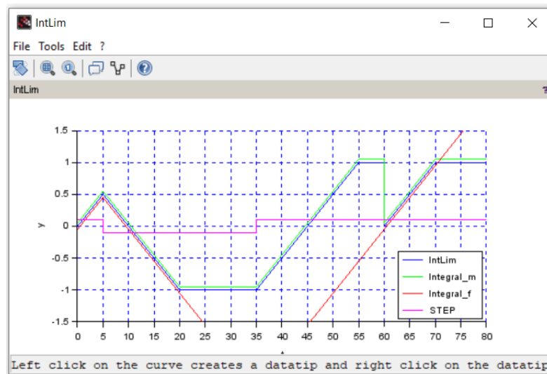
Figure 65 : Exemple de fenêtre graphique du programme de test associé au composant IntLim
