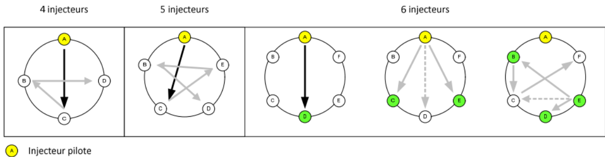
Figure 28 : Principe des commutations de jets, avec respect des calculs des efforts radiaux sur la roue PELTON
